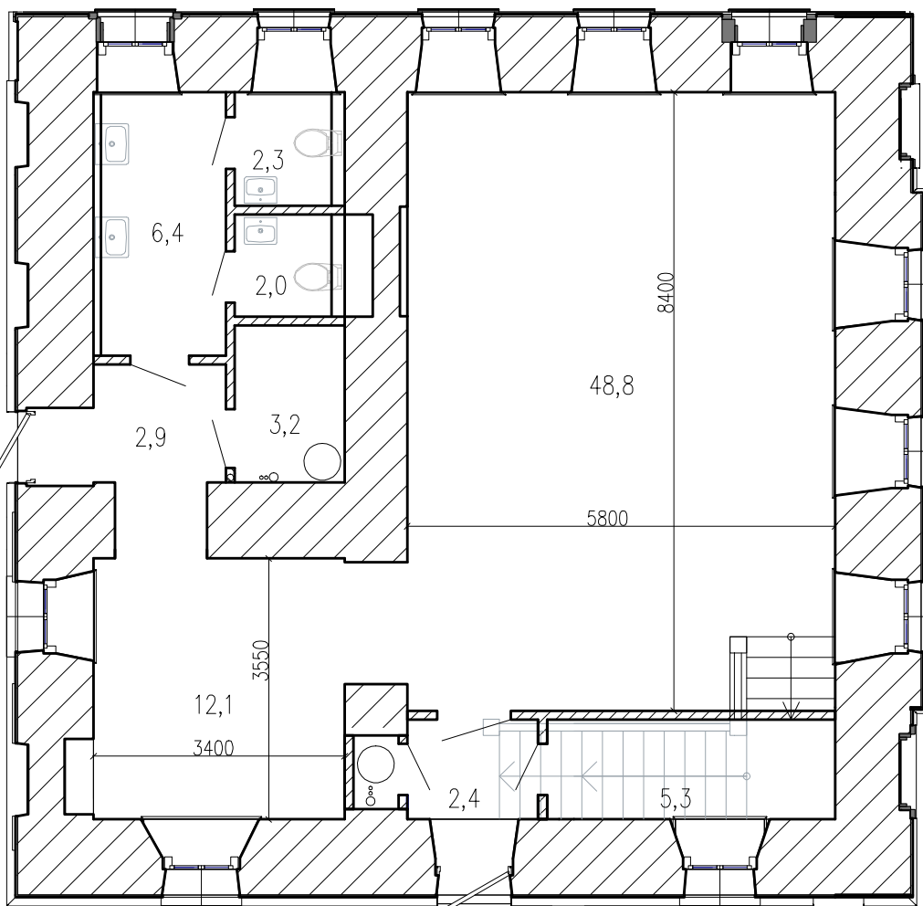
1 этаж
